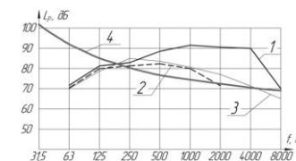
Рис. 1. Уровни звуковой мощности токарных станков
