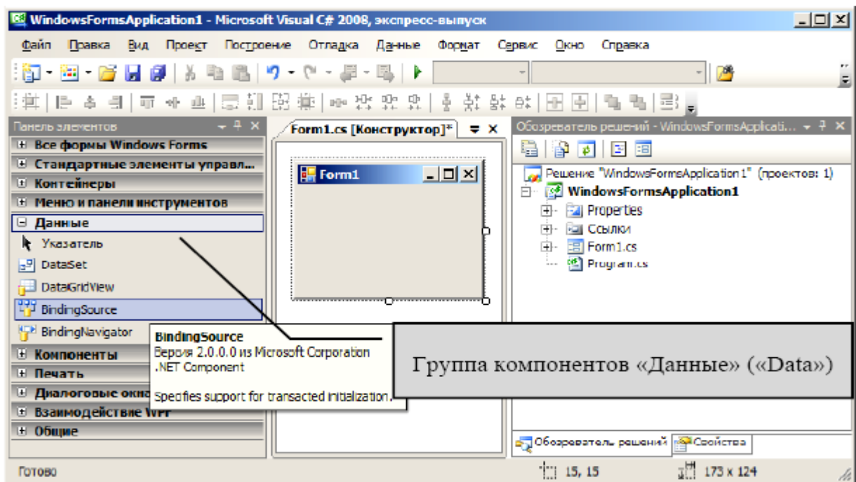
Рис. 39. Пустое приложение
