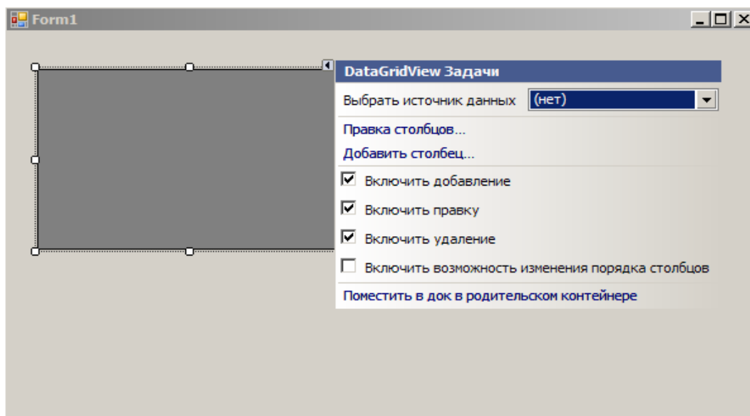
Рис. 46. Компонент DataGridView
