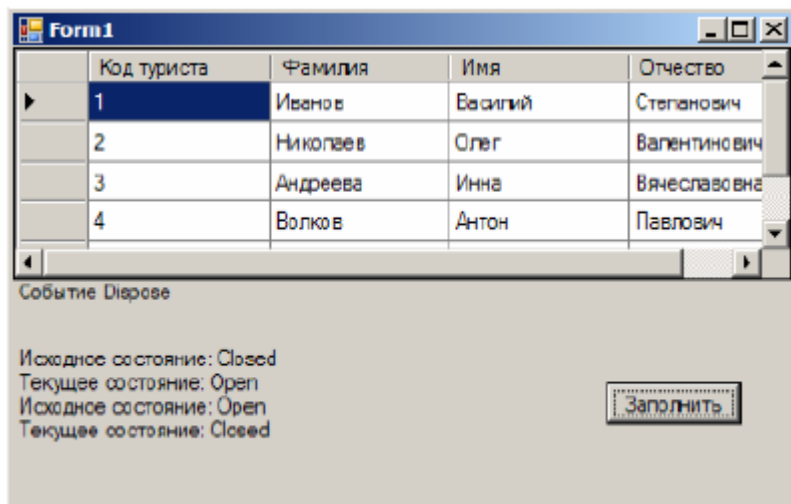
Рис. 61. Изменения состояния соединения с базой данных
